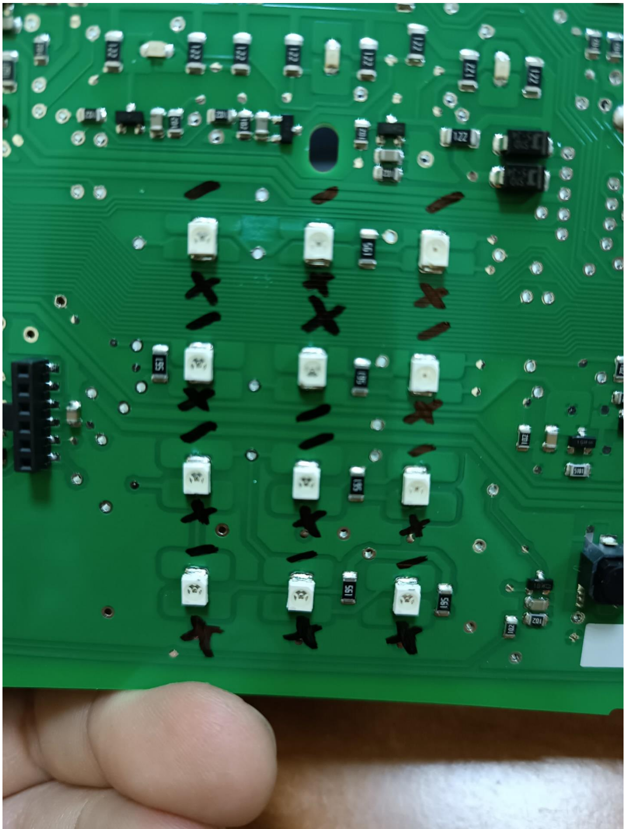
размечаем полярность диодов
