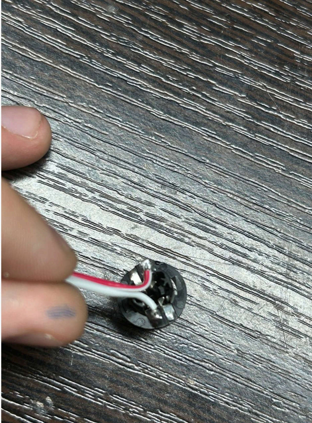
Провода припаиваем к цоколю таким образом.
