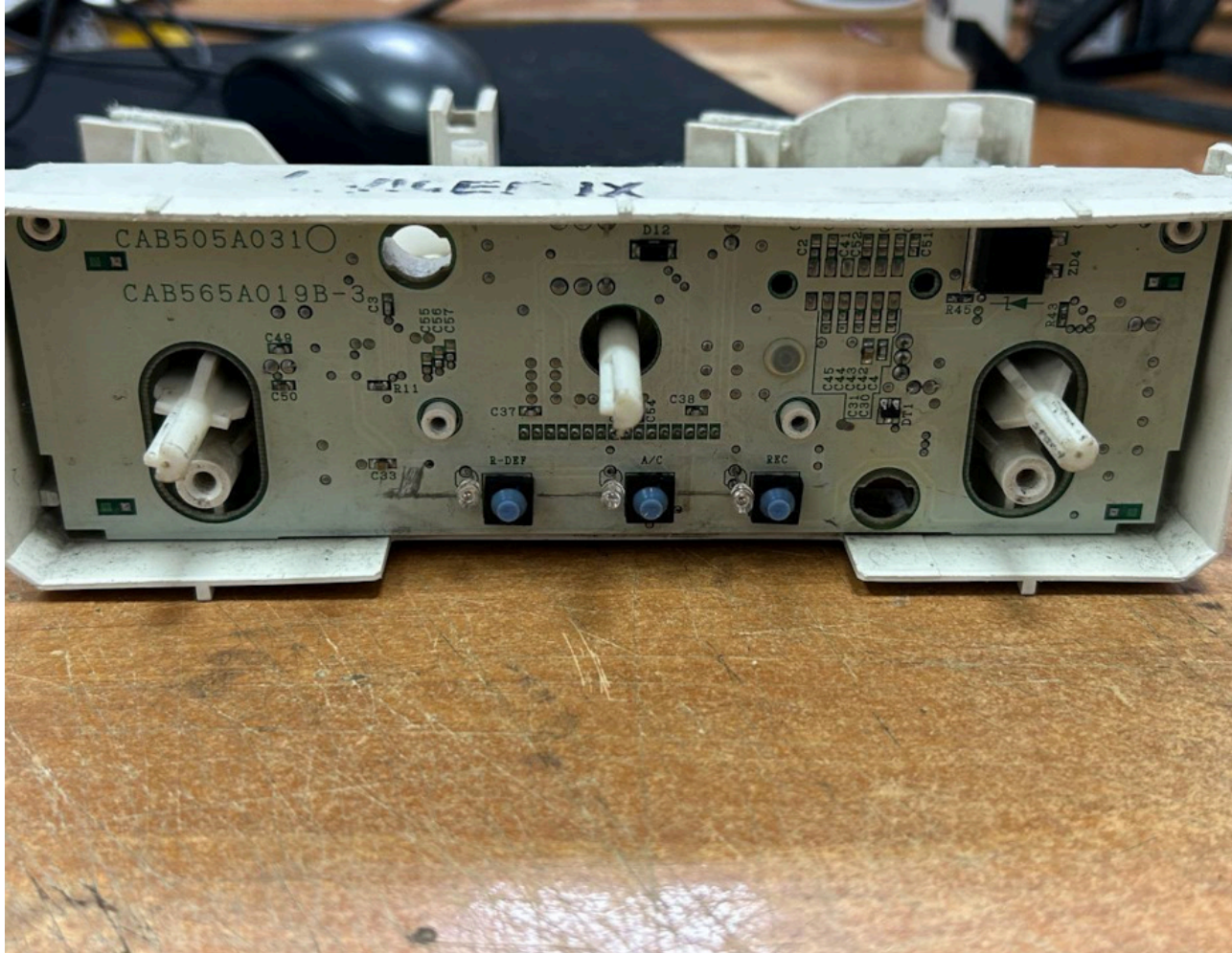
Вынимаем светорассеиватель и кнопки.
